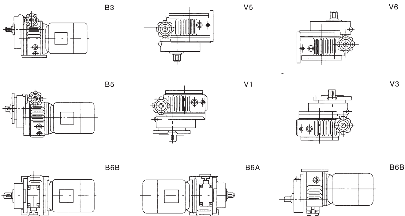
MB系列一配一级齿轮减速机的安装示例
