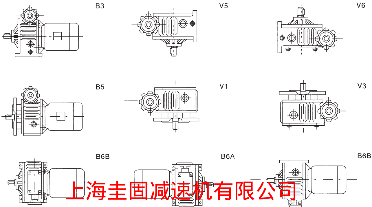
MB系列无级变速机基本型安装示例
