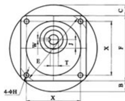
CVM22-50外形图
