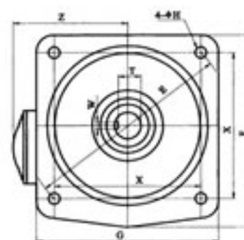
CV22-50外形图
