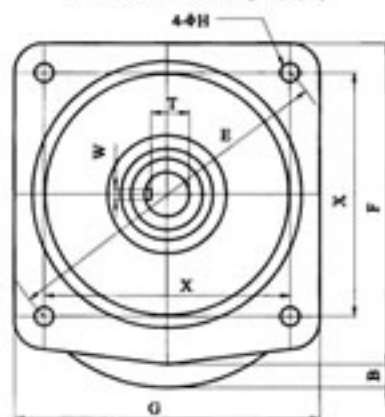
CVM22-50外形图
