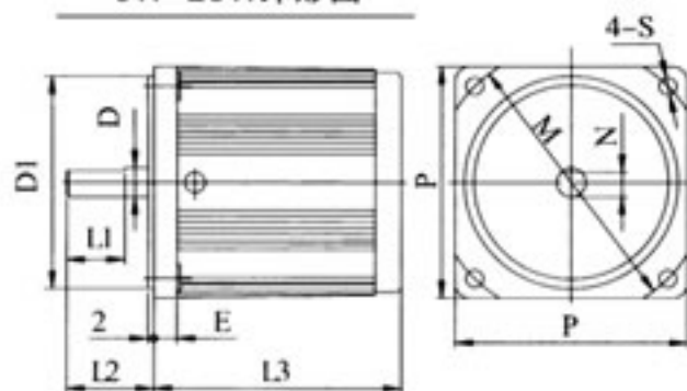
6W-25W外形图
