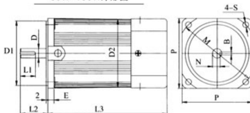
60W-180W外形图
