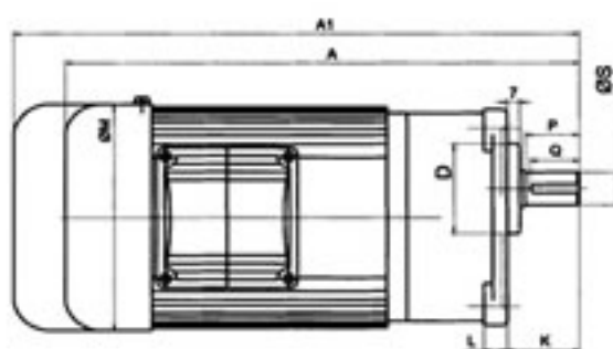
CV18外形图
