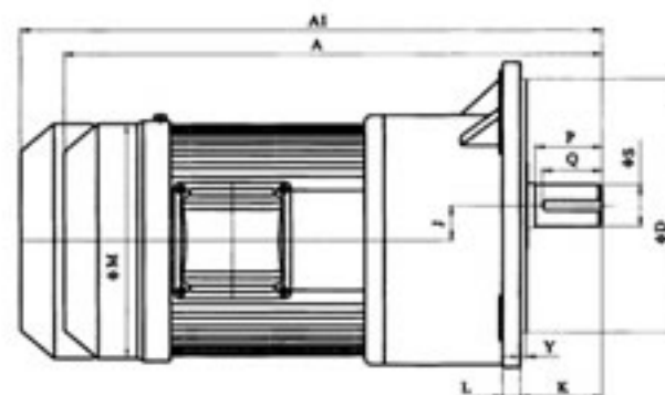
CV22-50外形图
